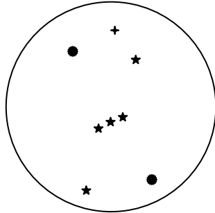
Orion
