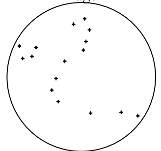
Dragen
