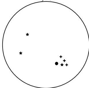
Tyren
