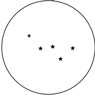
Kasiopeia
