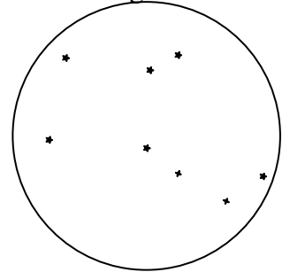
Pegasus
