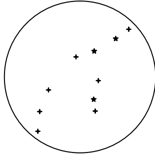
Persevs
