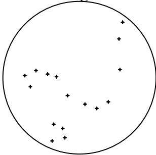
Dragen
