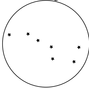
Karlsvogna
