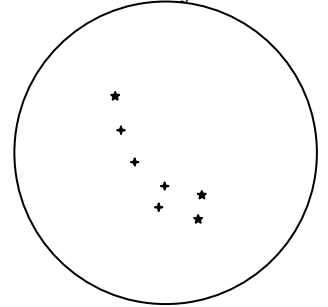
Lille bjørn
