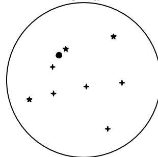
Ørna
